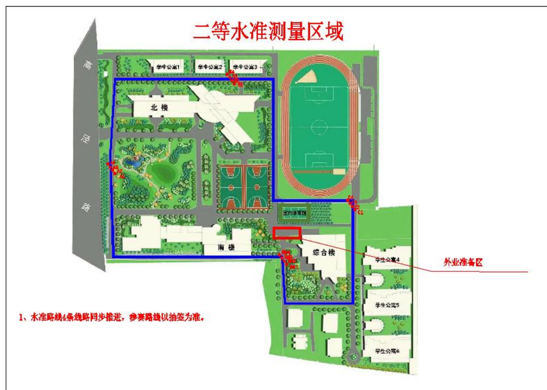
图 3 二等水准区域及相关空间示意图
