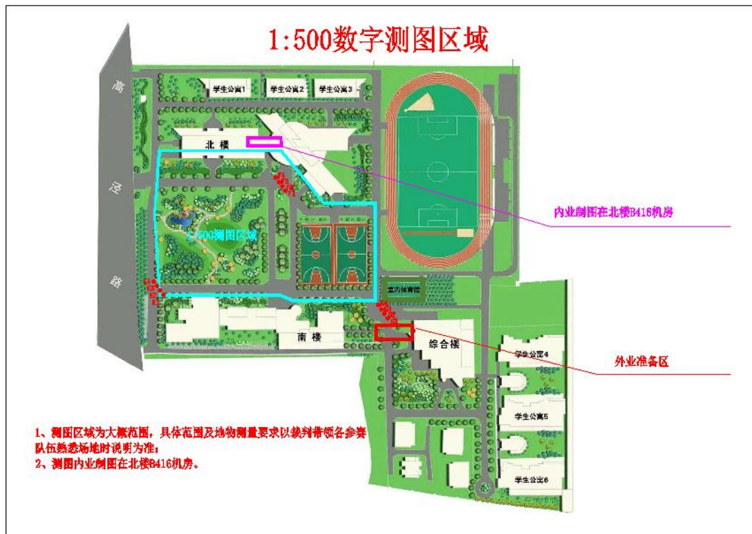
图 2 1: 500 数字测图区域及相关空间示意图
