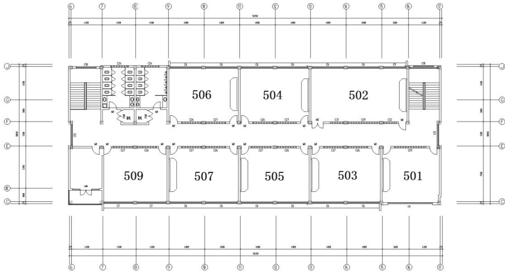
17号楼平面图
